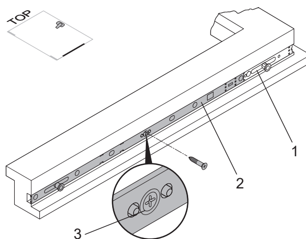
Средняя блокада М/МК (устанавливается по горизонтали)
