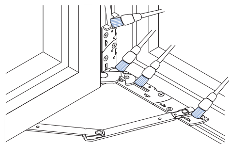
Кронштейн (Створка/Рама), Петля на раму, Шина петли створки
