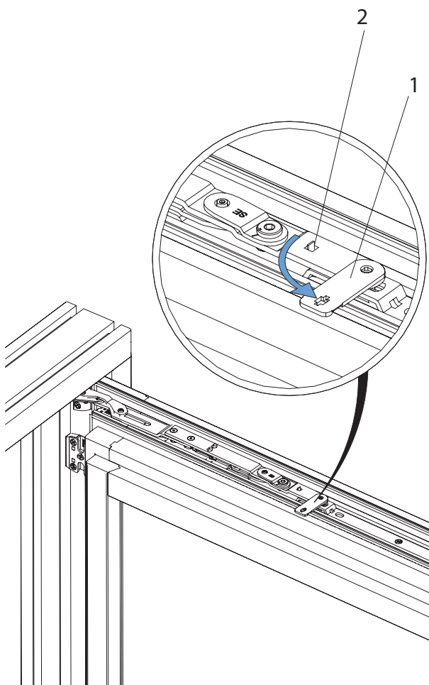
Снятие створки
